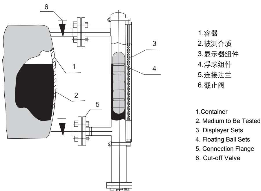
图三 安装图
